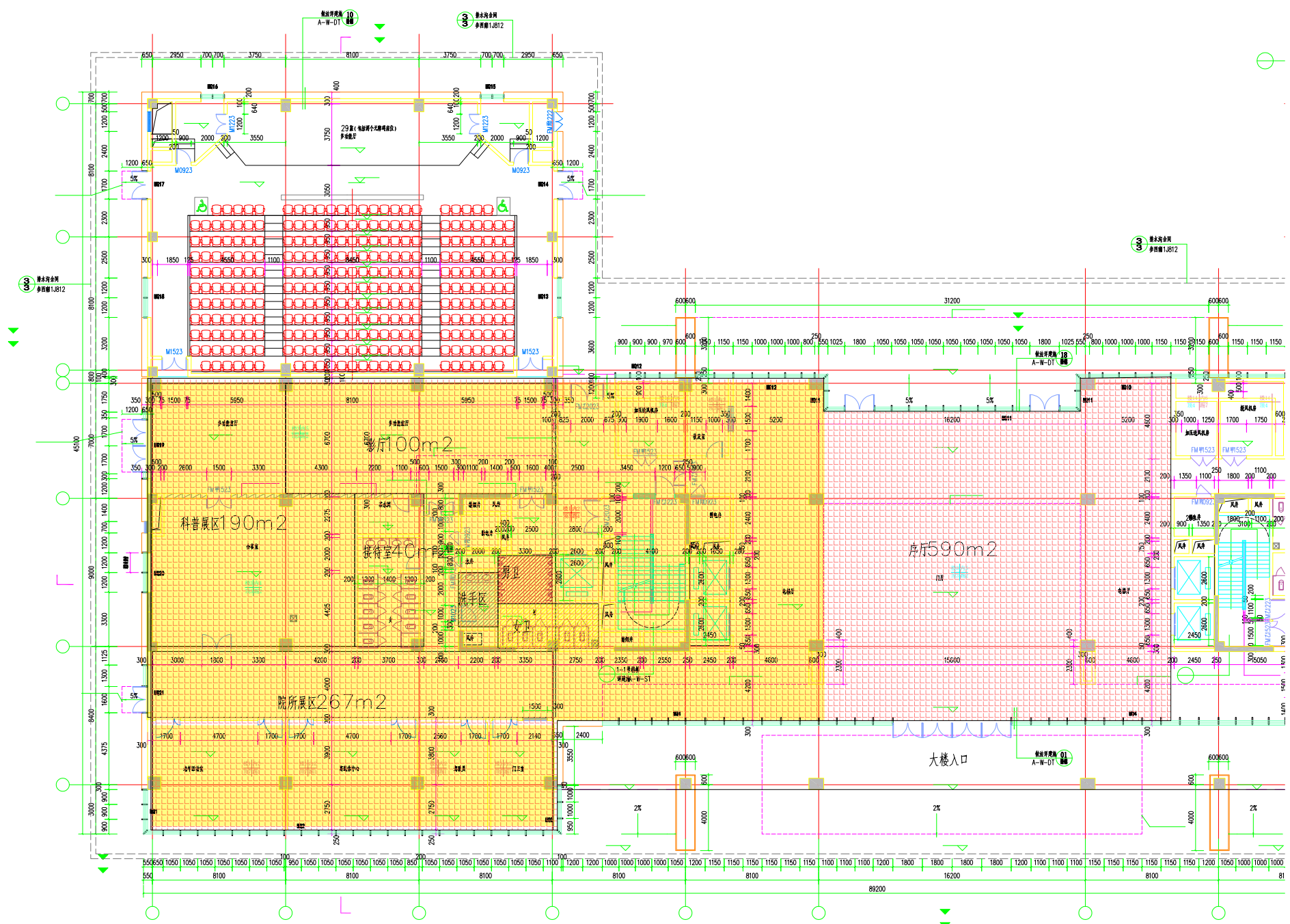
科研办公楼 (1号楼) 首层平面图 1:100
